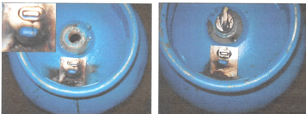
Fig. Capa metálica com ID 103M e capa plástica ID 103G coladas ao botijão
