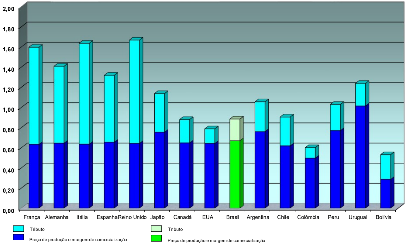
2.6 - Preços do Óleo Diesel ao Consumidor, com Tributos (US$/Litro) em jan/19 Brasil, América do Sul e OCDE
