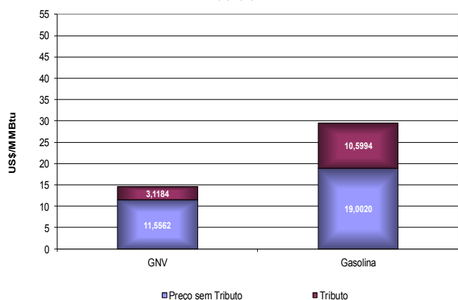
Comparativo de Preços entre Gás Natural Veicular e Gasolina em São Paulo - maio/2016
