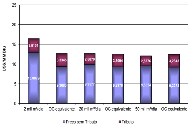
Comparativo de Preços entre Gás Natural Industrial e OCA1 em São Paulo - maio/2016
