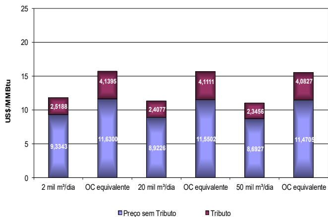
Comparativo de Preços entre Gás Natural Industrial e OCA1 na Bahia - março/2017
