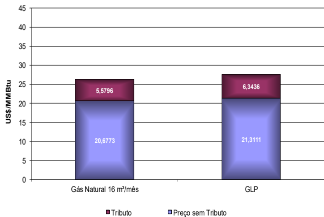
Comparativo de Preços entre Gás Natural Residencial e GLP na Bahia - março/2017
