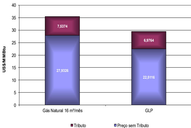
Comparativo de Preços entre Gás Natural Residencial e GLP em São Paulo - março/2017
