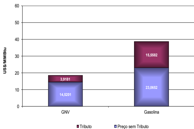
Comparativo de Preços entre Gás Natural Veicular e Gasolina no Rio de Janeiro - março/2017
