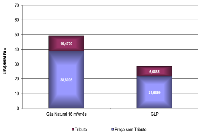
Comparativo de Preços entre Gás Natural Residencial e GLP no Rio de Janeiro - março/2017
