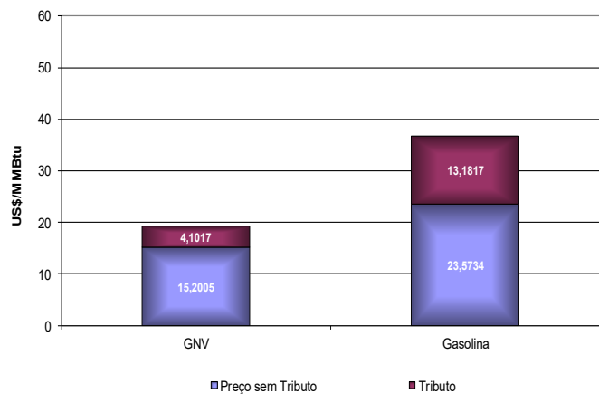
Comparativo de Preços entre Gás Natural Veicular e Gasolina na Bahia - março/2017
