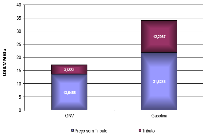
Comparativo de Preços entre Gás Natural Veicular e Gasolina em São Paulo - março/2017
