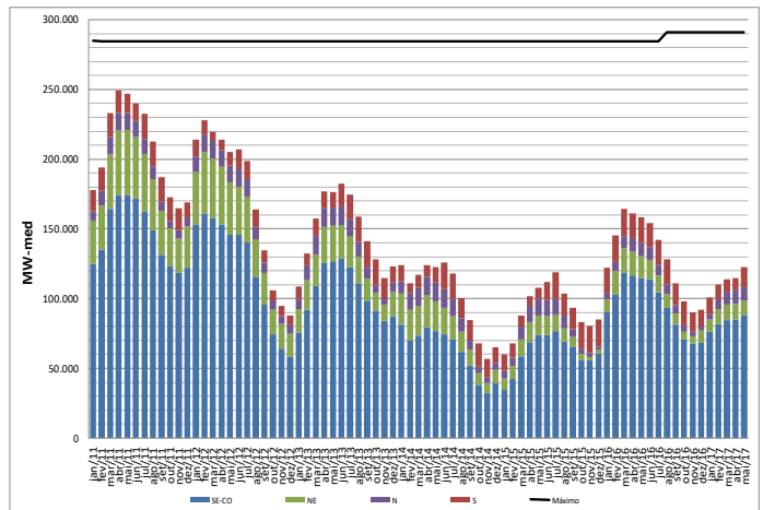
Em MWh/mês
