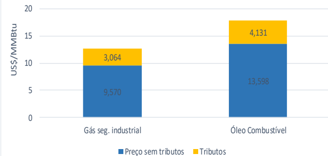
Comparativo de preços entre gás natural para segmento industrial (20.000 m 3 /d) e óleo combustível em São Paulo - junho/2018
