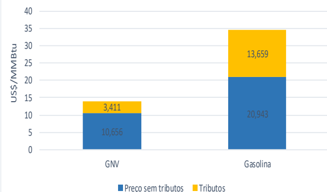
Comparativo de preços entre GNV e gasolina em São Paulo - junho/2018
