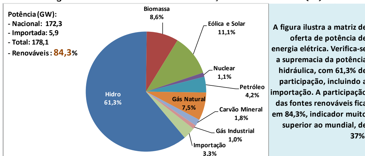
Figura 4: Oferta de Potência de Geração Elétrica – 2019 (%)
