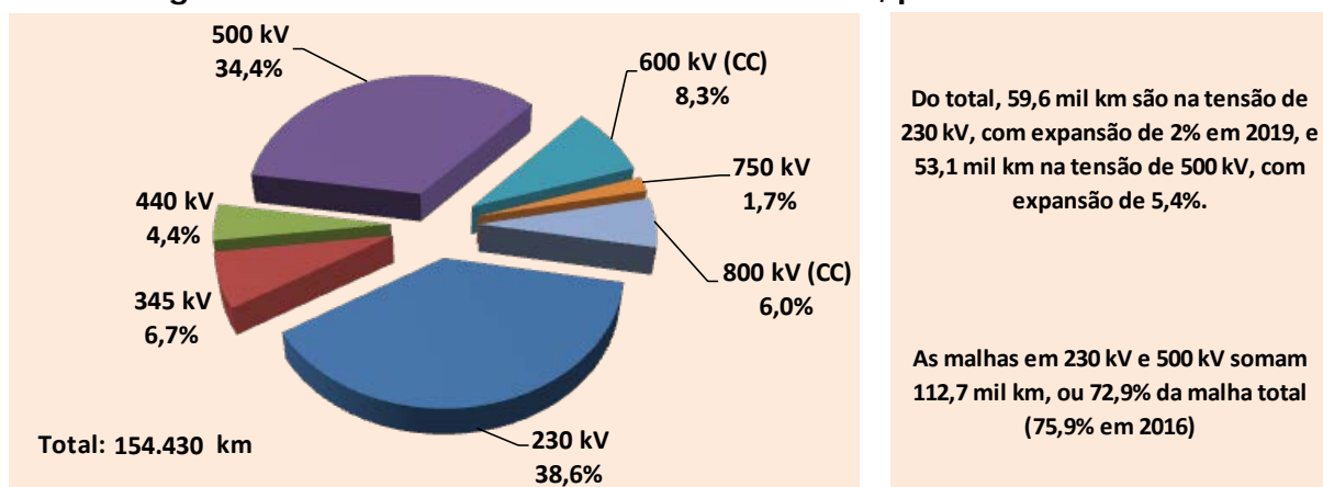
Figura 5: Estrutura da Malha de Transmissão, por Tensão - 2019
