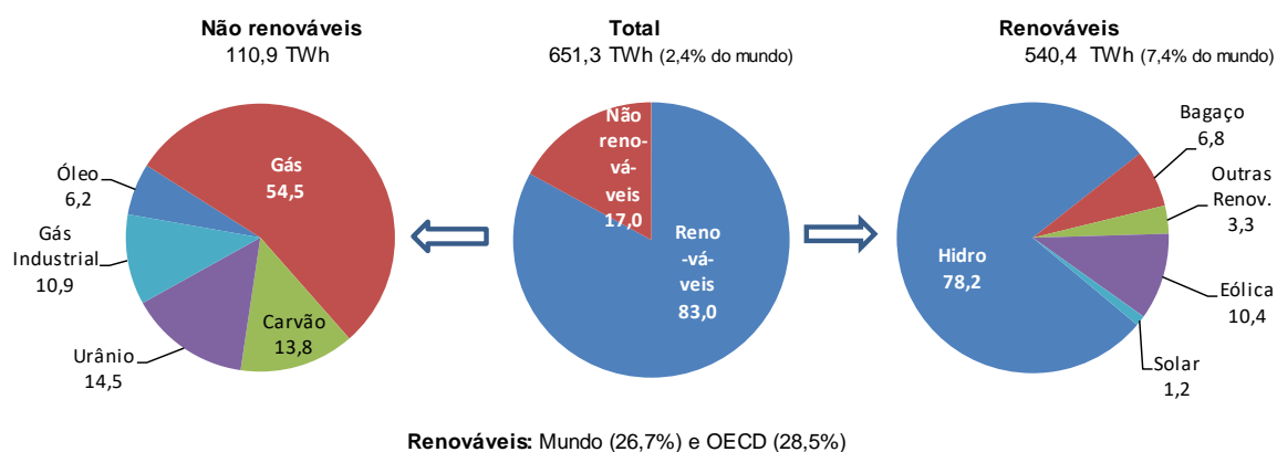
Figura 3: Oferta Interna de Energia Elétrica - 2019 (%)
