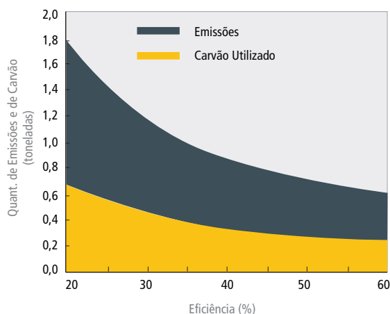
Figura 10 – Relação entre eficiência de usinas térmicas e emissões de poluentes
