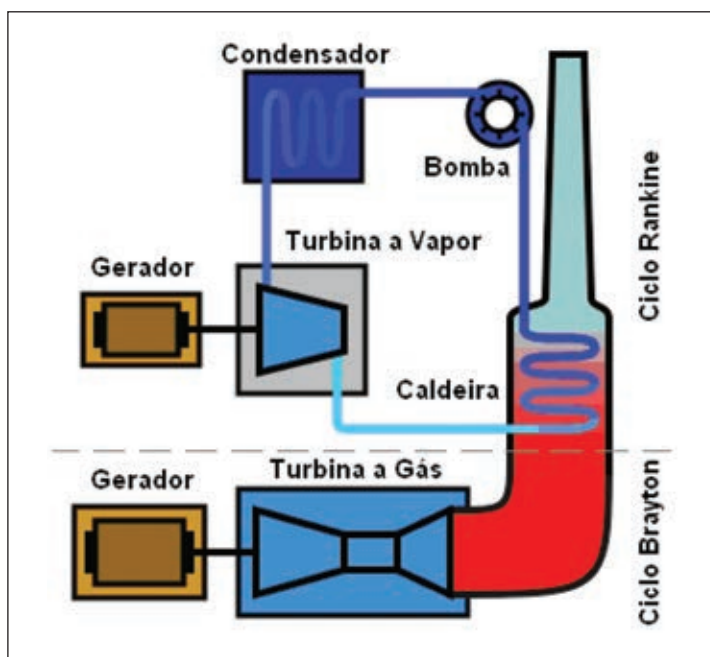
Figura 6 – Diagrama esquemático do ciclo combinado
