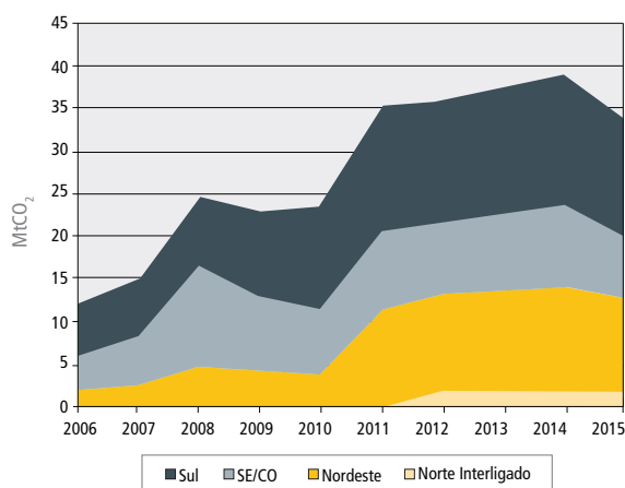
Figura 3 - Estimativas das emissões de CO 2 (2006 – 2015)
