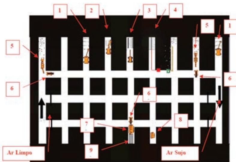
Figura 4 – Representação esquemática de mineração de câmaras e pilares
