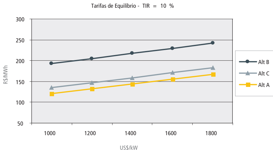
Figura 12 – Comparação das tarifas de acordo com o tipo de carvão para uma mesma Taxa Interna de Retorno
