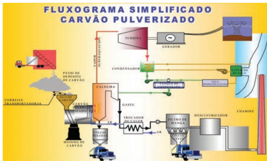
Figura 7 – Esquema simplificado de usina a carvão pulverizado
