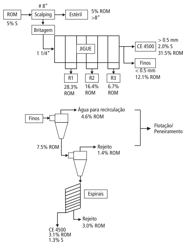
Figura 9 – Circuito típico de beneficiamento nos lavadores de Santa Catarina
