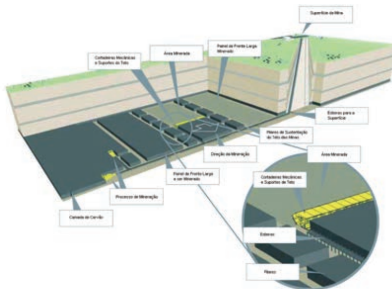
Figura 3 – Operação de uma mina subterrânea
