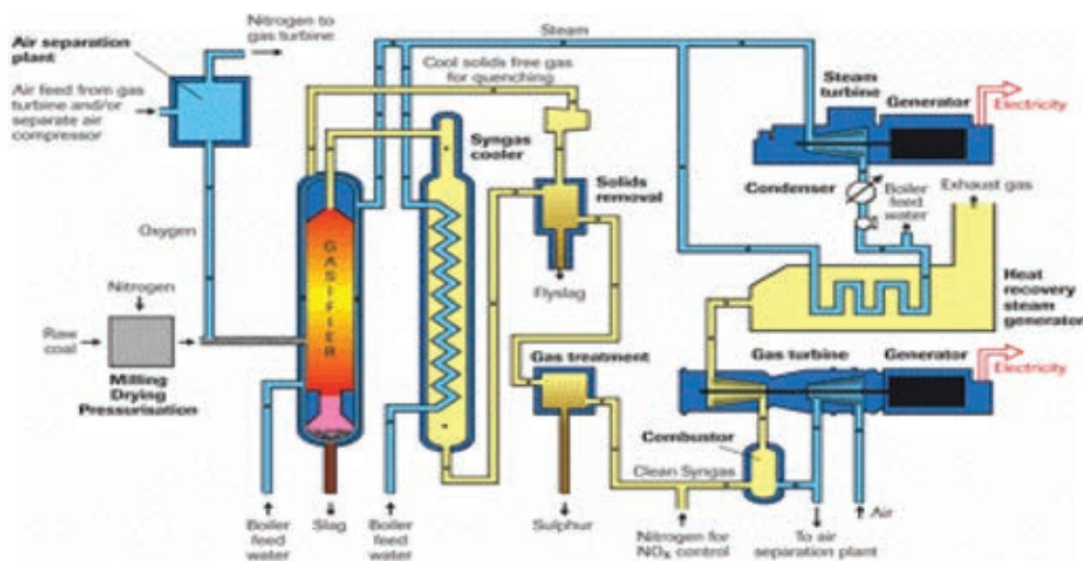
Figura 9 – Esquema do sistema de gaseificação integrada com ciclo combinado
