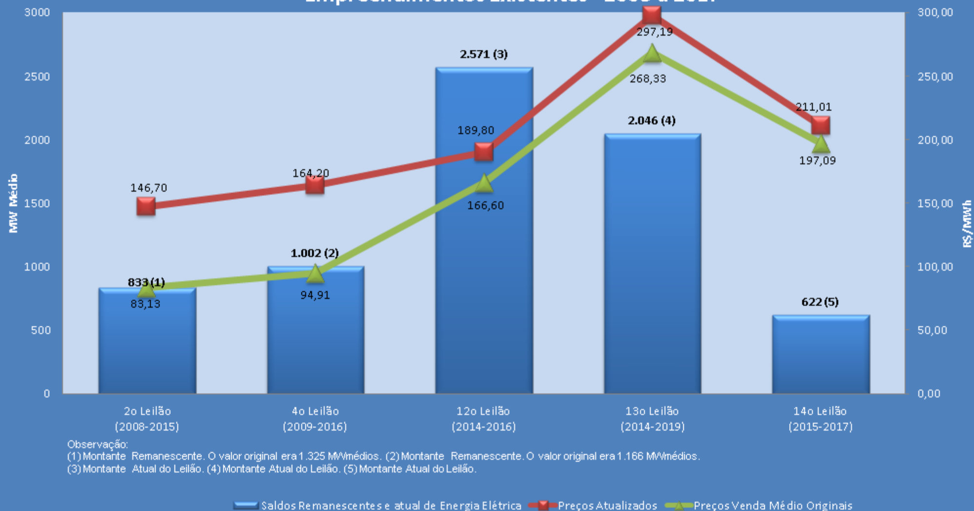
Figura 6 - Montantes e Preços Adjudicados / Valores atualizados pelo IPCA até Agosto/2015
