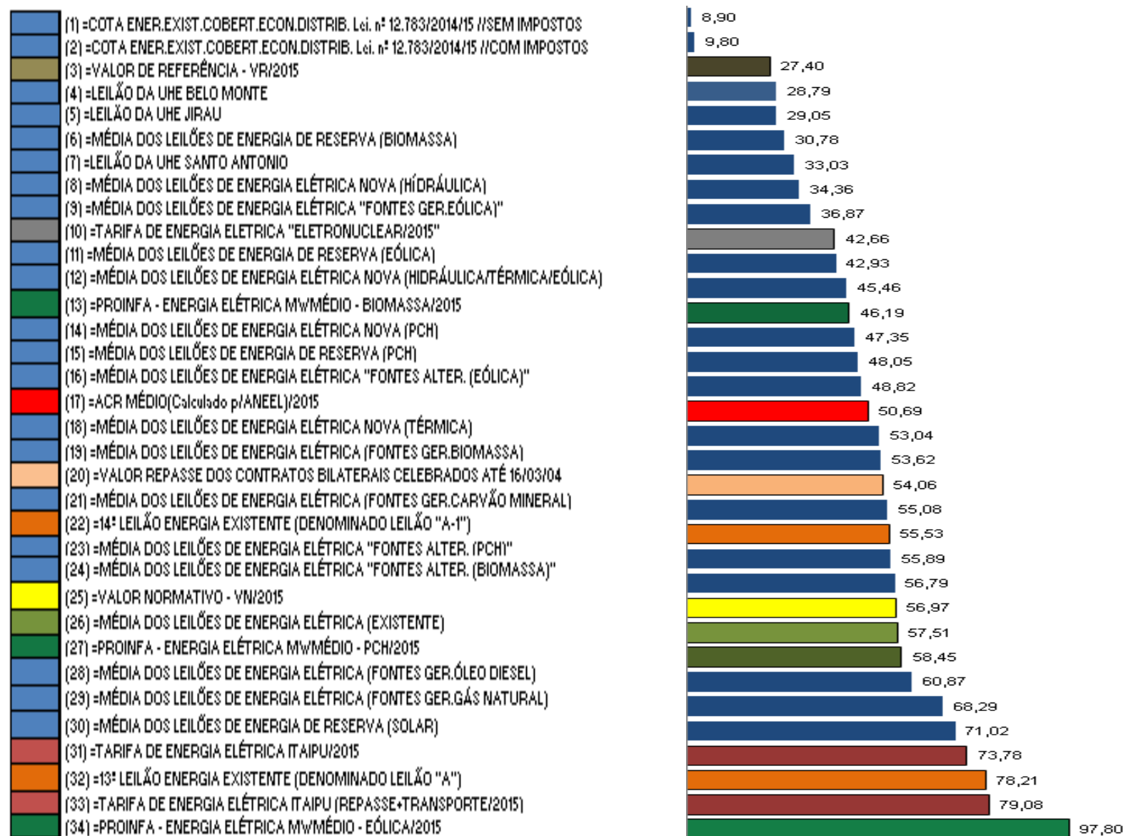
Figura 2 - Preço dos Contratos de Suprimento/Valores em US$/MWh 1US$=R$ 3.80
