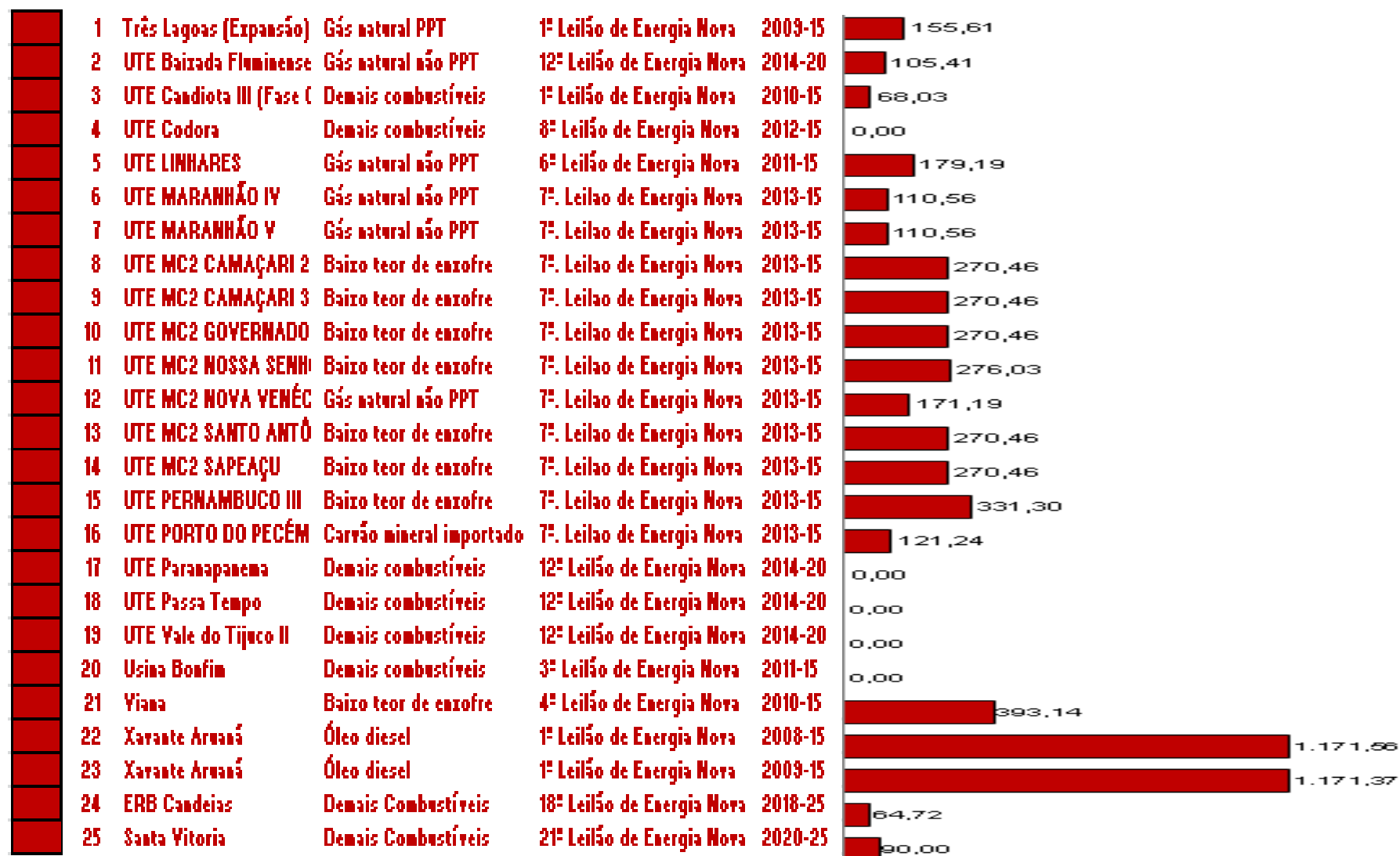
Figura 5 – CVU Leilões de Energia Elétrica/Valores em R$/MWh
