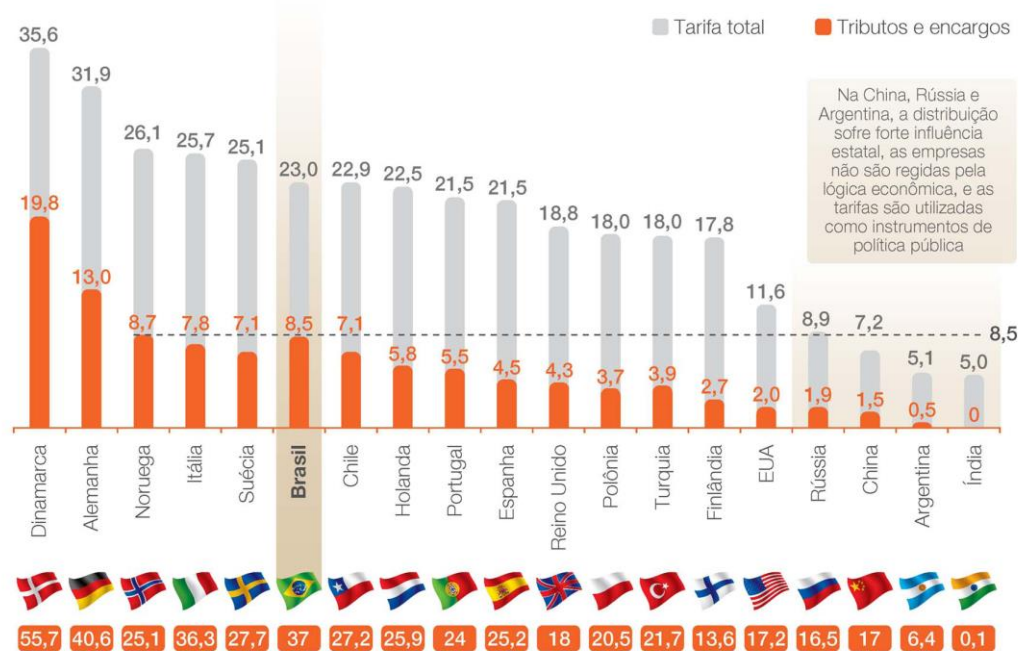
Tarifa residencial média de energia elétrica, US$/kWh, 2010
