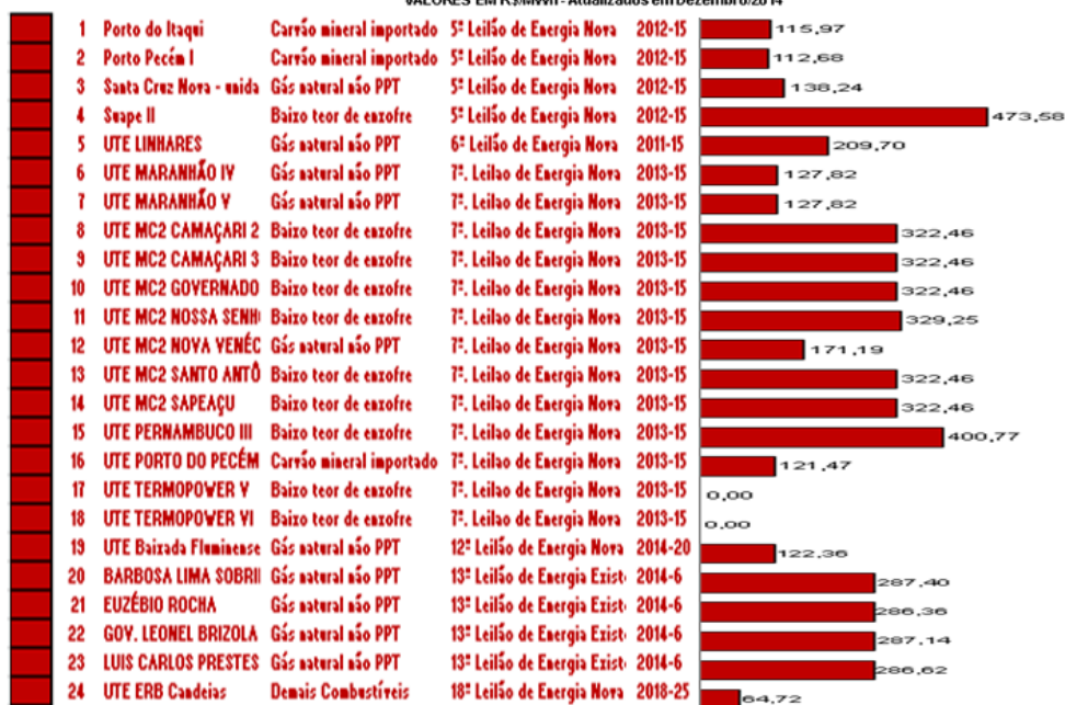
Figura 5 - CVU 5º 6º 7º 12º LEN e 13º LEE Leilão de Energia Nova/Existente Valores em R$/MWh
