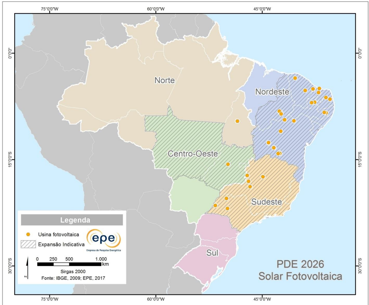
Figura 7 – Localização da expansão solar fotovoltaica planejada no PDE 2026
