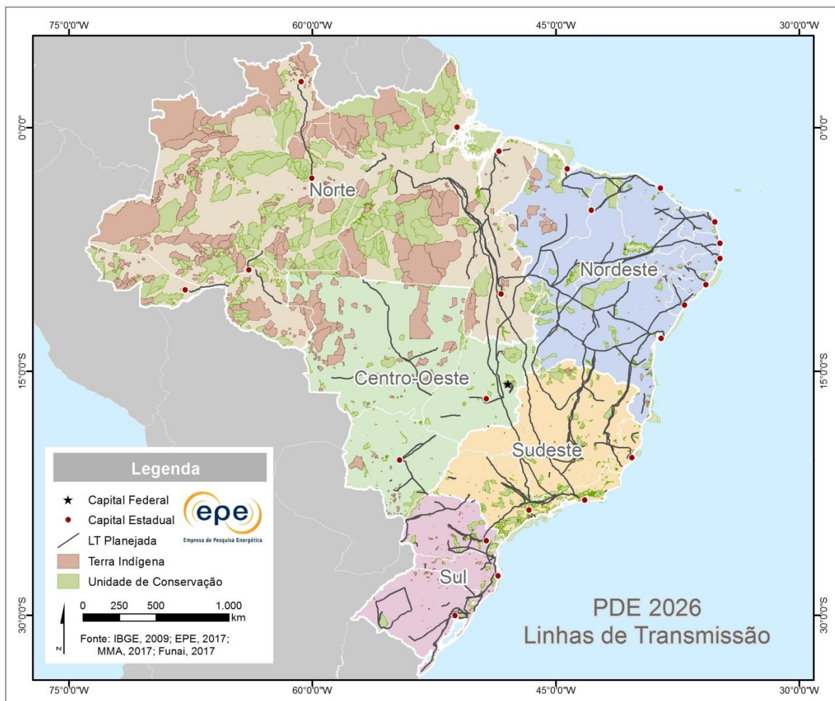
Figura 8 – Linhas de transmissão previstas no PDE 2026 e áreas legalmente protegidas
