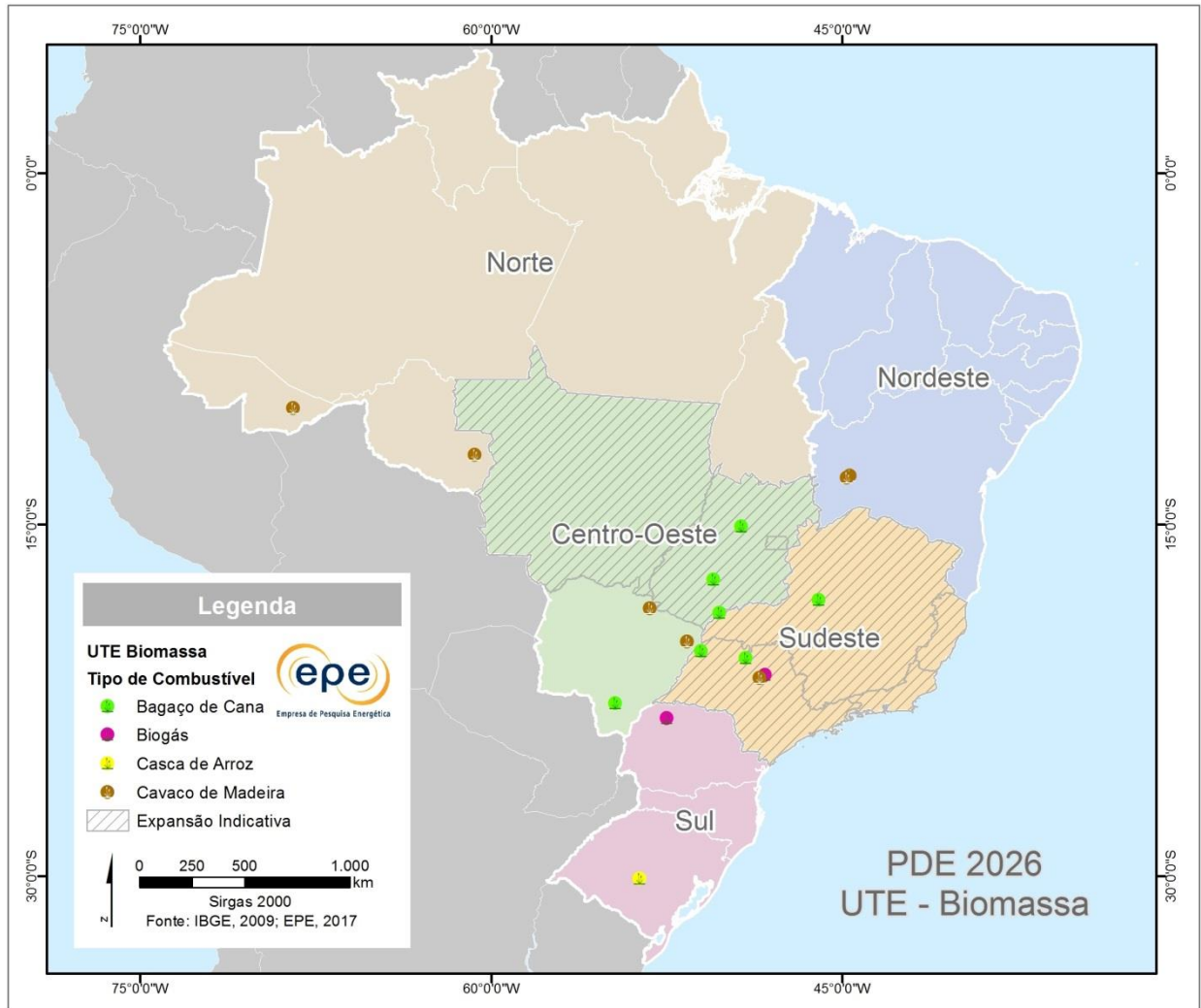
Figura 5 – Localização da expansão termelétrica a biomassa planejada no PDE 2026
