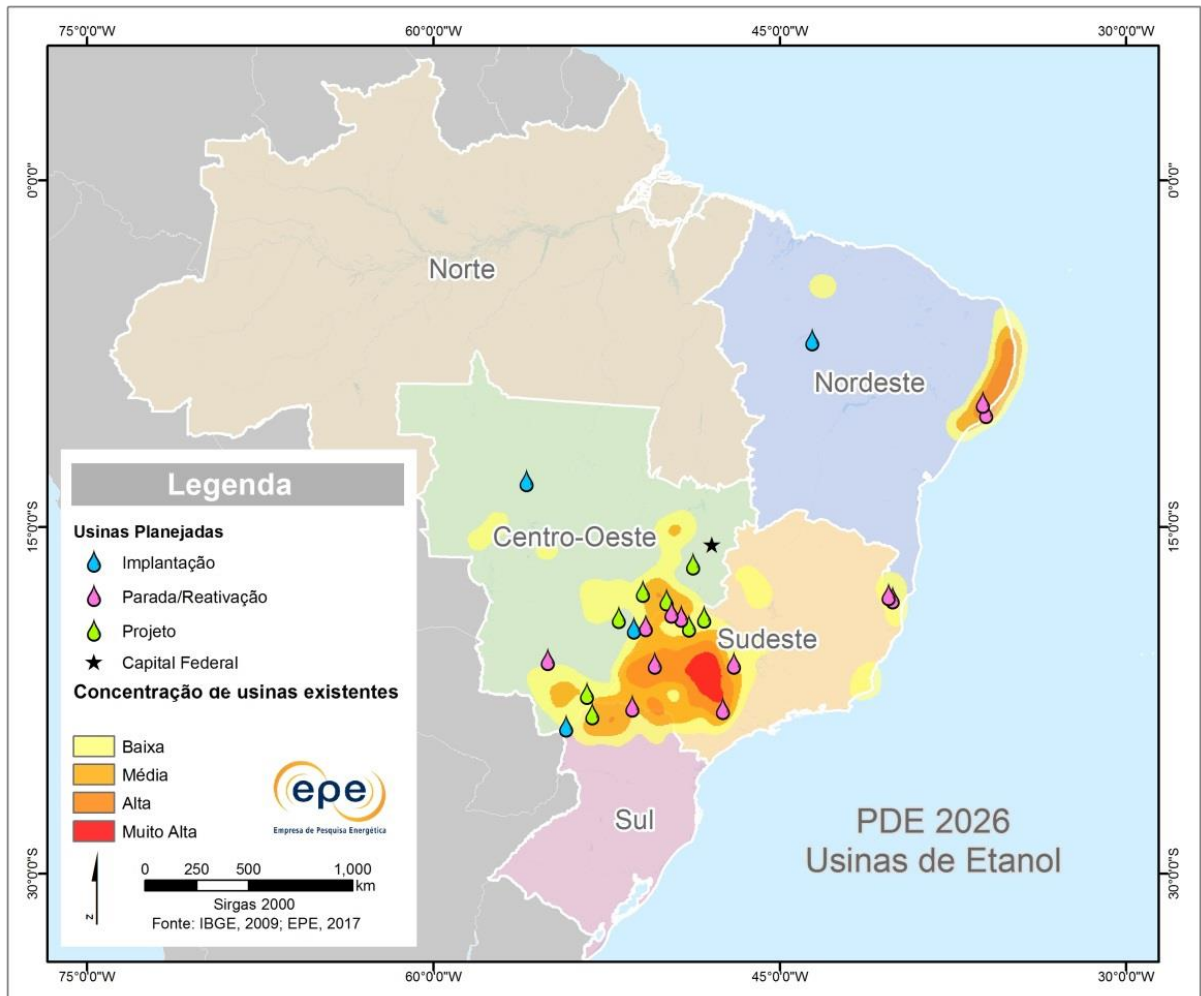
Figura 10 – Concentração de usinas existentes e localização das usinas planejadas
